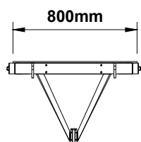
Vista frontale modulo ponte Deck Module Front View
