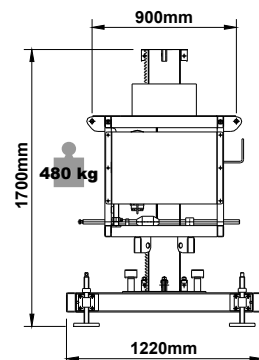
Dettagli gruppo di sollevamento Drive unit details
