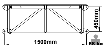
Dettagli modulo ponte Deck module details
