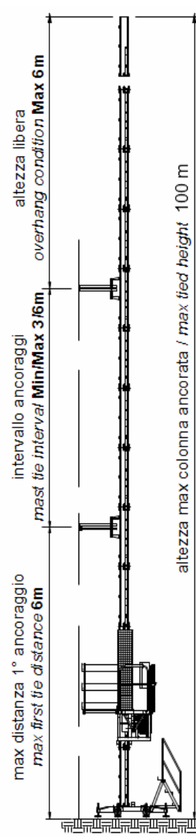
Dettagli ancoraggi Tie details
